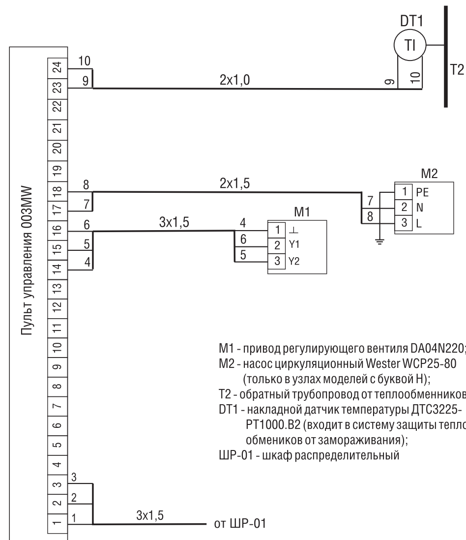
Рисунок 6 Схема электрическая подключений смесительного узла
